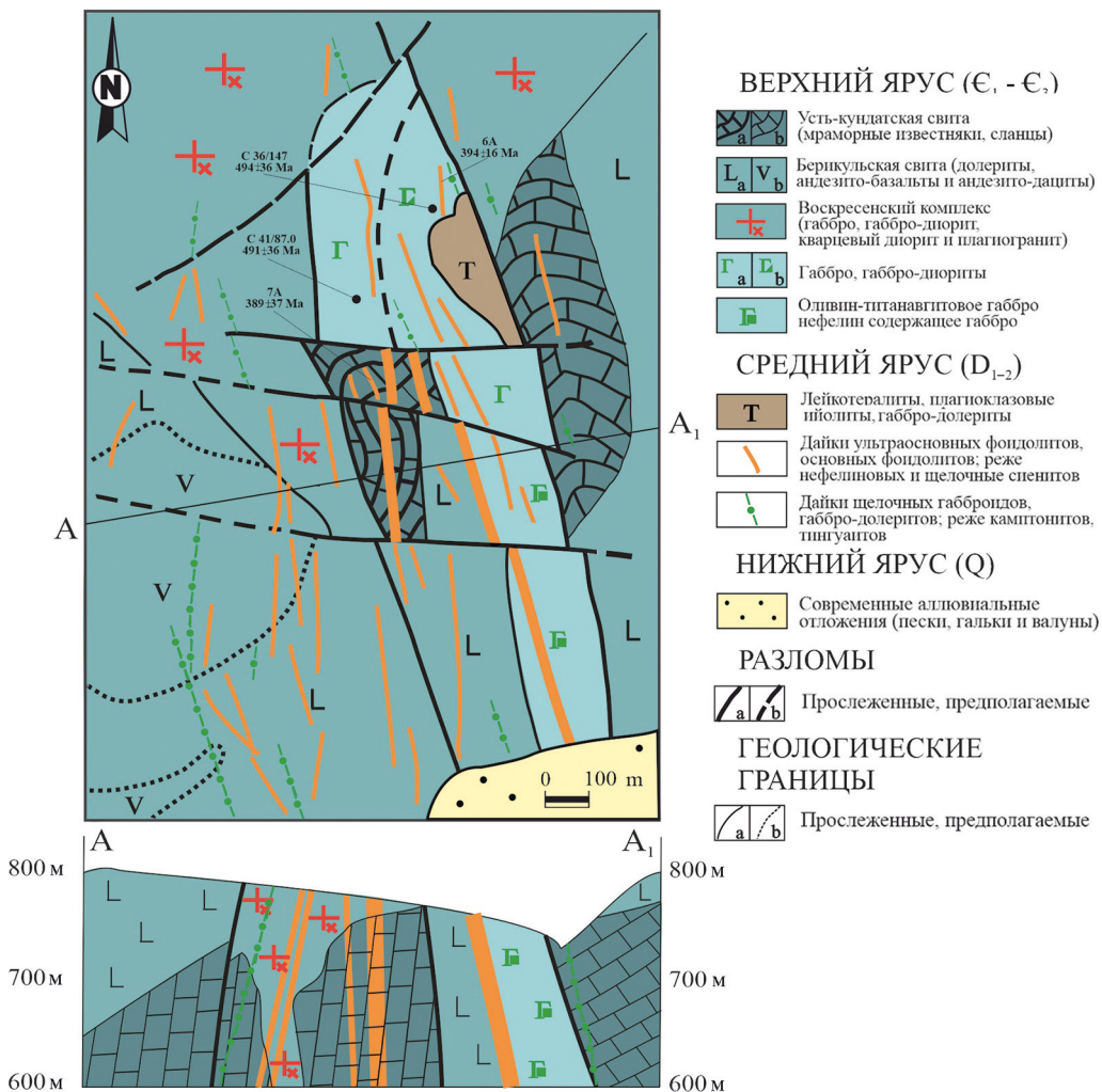
Рис. 2. Схема геологического строения и разрез по линии А-А 1 Университетского плутона в масштабе 1:5000 по (Есин и др., 1987; Осипов и др., 1989) с дополнениями авторов
