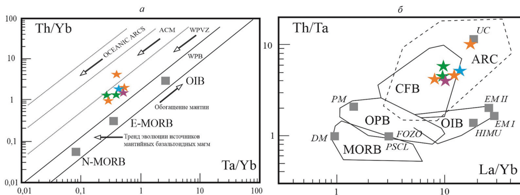
Рис. 7. Соотношения несовместимых элементов в породах Университетского плутона:
