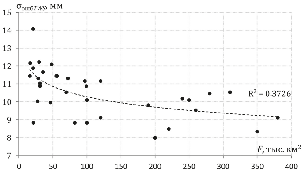
Рис. 1. Ошибка определения TWS за холодный период при различной площади водосбора (по данным GRACE для рек ЕЧР)
