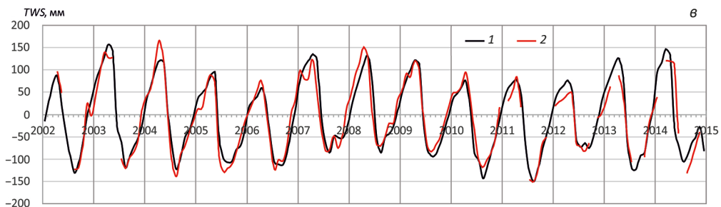
Рис. 3. Аномалии влагозапасов в бассейнах рр. Сев. Двины (а), Печоры (б), Мезени (в) по результатам моделирования на основе модели ECOMAG (1) и по данным спутников GRACE (2)
