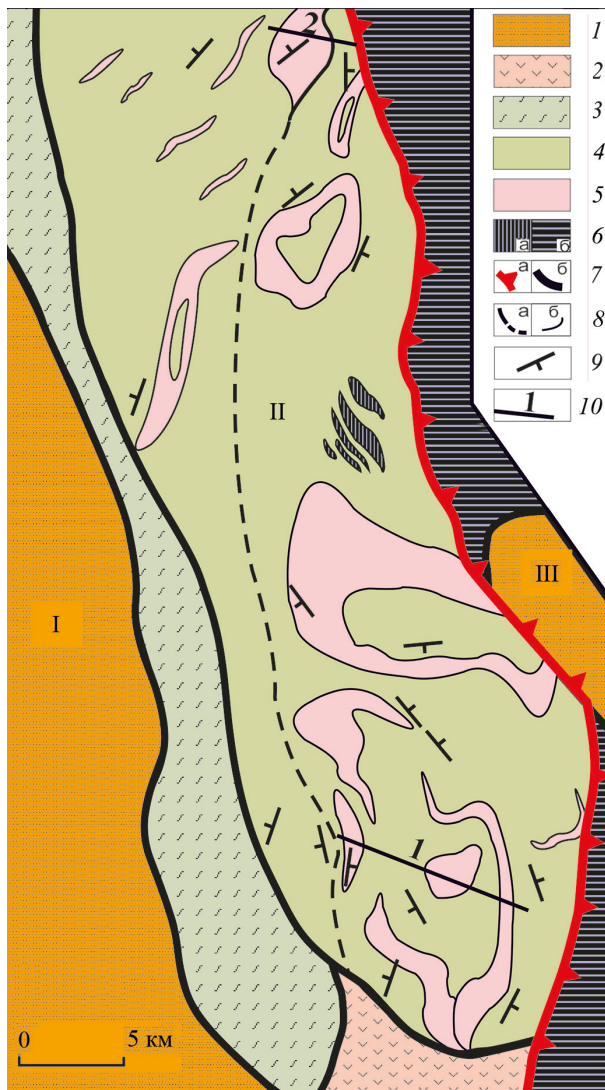
Рис. 2. Структурная схема южной части зоны (антиформы) Уралтау и ее обрамления
