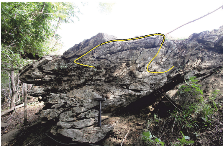
Рис. 7. Складки с крутопадающими шарнирами F_4 , верховья р. Губерля (а), колчановидная складка F_1 , верховья р. Дергамыш (б)
