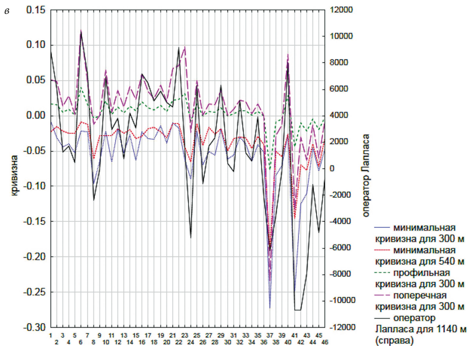
Рис. 1. Распределение разных типов сообществ в зависимости от характеристик рельефа: а — высота, м; б — освещенность; в — показатели кривизны поверхности и их производная (оператор Лапласа). По оси абсцисс — нумерация синтаксонов, соответствующая номерам в прил. 3.1
