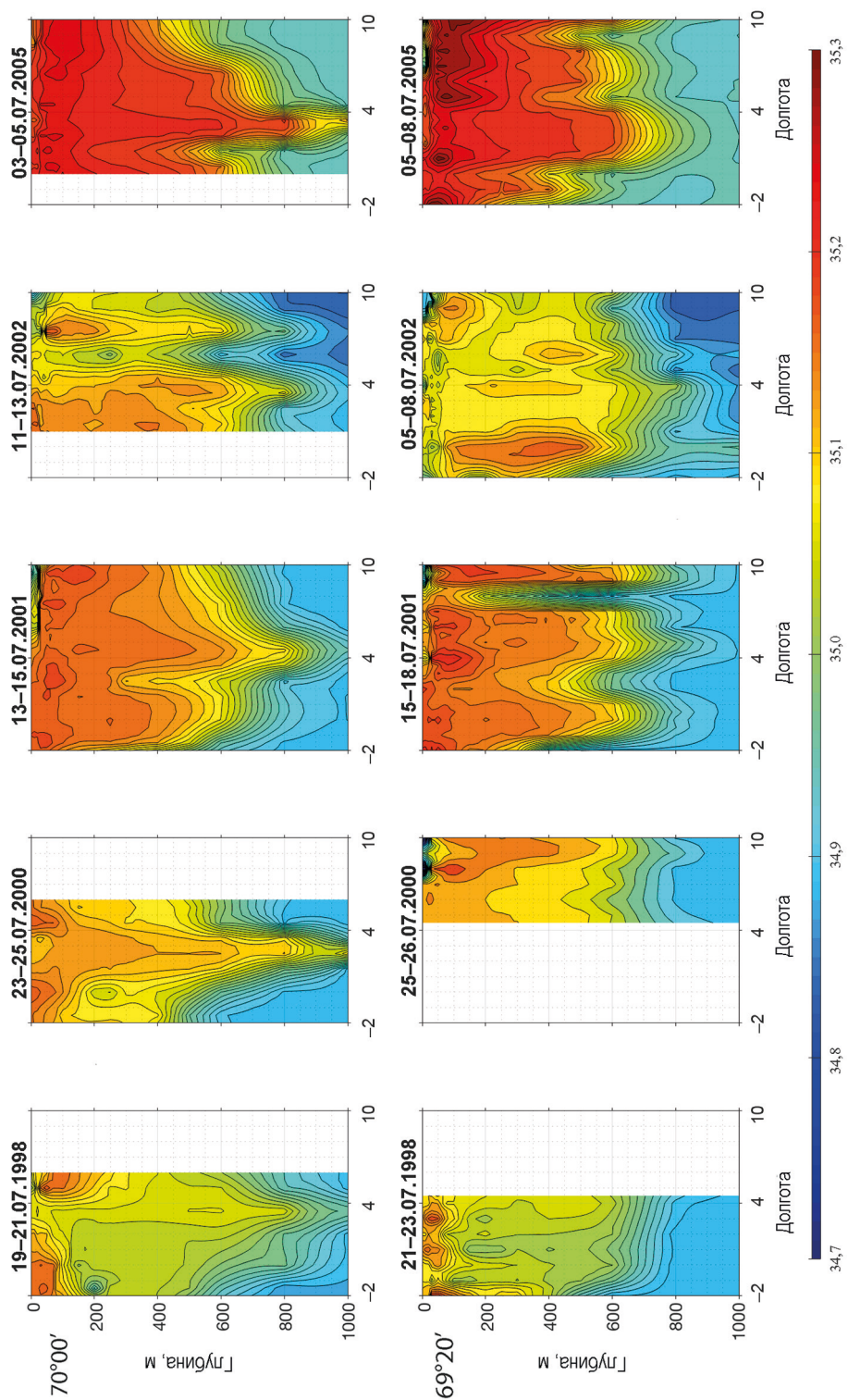
Рис. 4. Соленость воды, измеренная на разрезах по 70°00' и 69°20' с. ш. в июле 1998, 2000, 2001, 2002 и 2005 гг.
