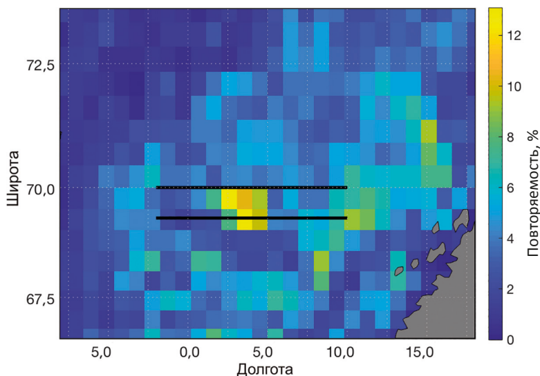
Рис. 2. Повторяемость антициклонических вихрей (Faghmous et al., 2015) Параллельные отрезки — расположение гидрологических разрезов вдоль 69°20' и 70°00' с. ш.
