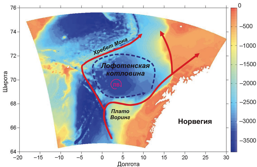
Рис. 1. Топографическая карта Лофотенской котловины
